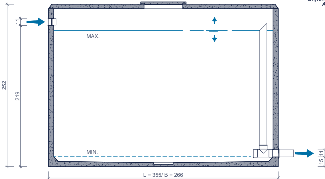
doorsnede coupe
